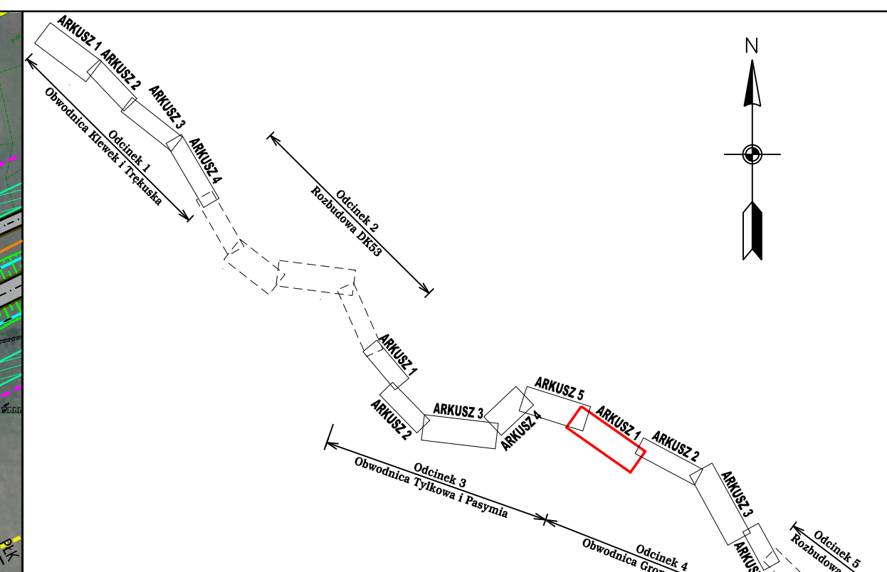
SCHEMAT ROZMIESZCZENIA ARKUSZY WARIANT NIEBIESKI
